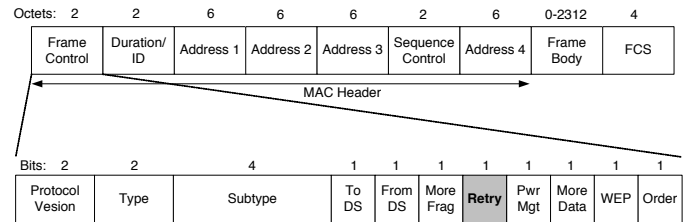
Fig. 6. General IEEE 802.11 MAC layer frame format
